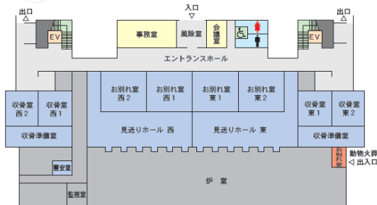
1 階平面図
